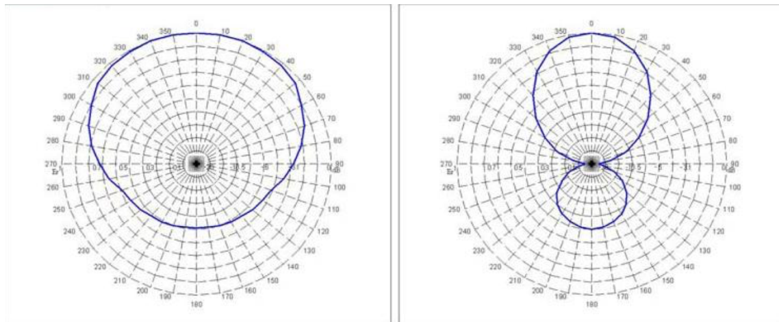
DIAGRAMA DE RADIACIÓN HORIZONTAL
